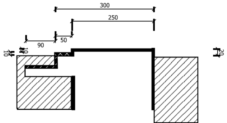
Coupe de principe
